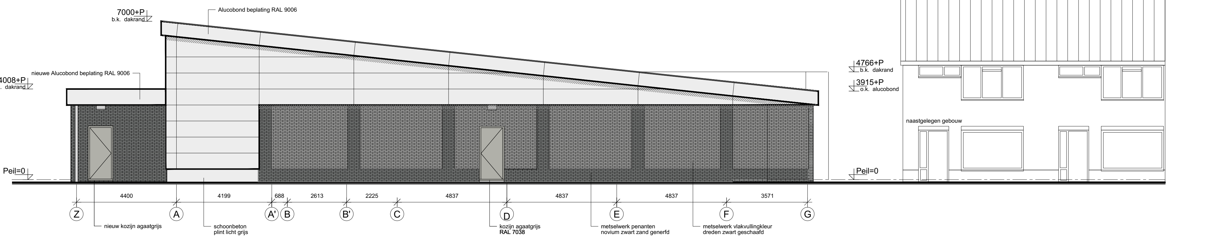
- Linkerzijgevel (Anjelierstraat) -
